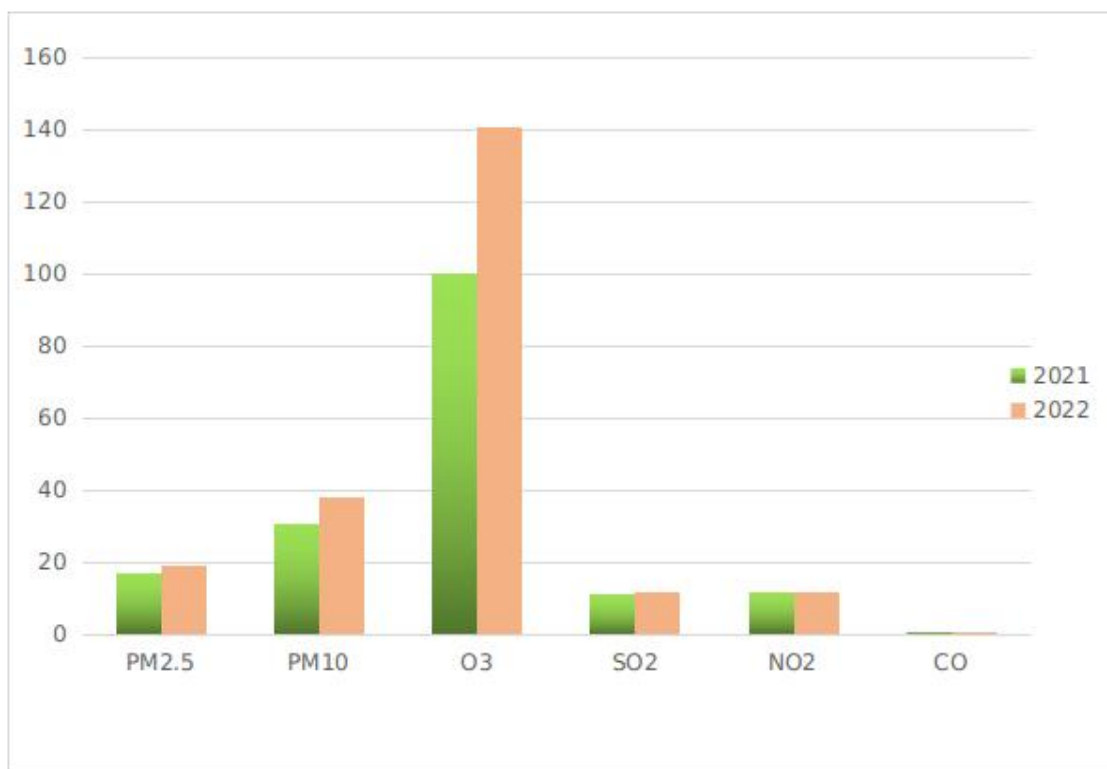
图1 我市2021年7月与2022年7月空气质量对比图
