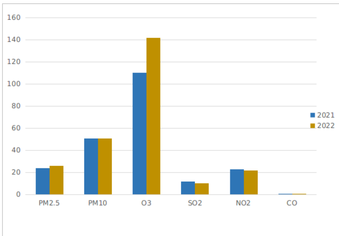
图1 我市2021年4月与2022年4月空气质量对比图
