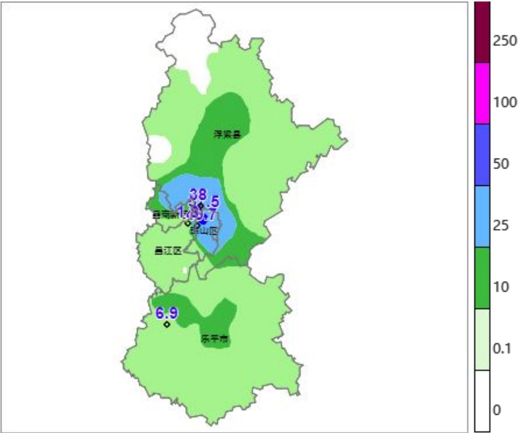
图 1 过去 3 小时(21:40-00:40)累计雨量实况图
