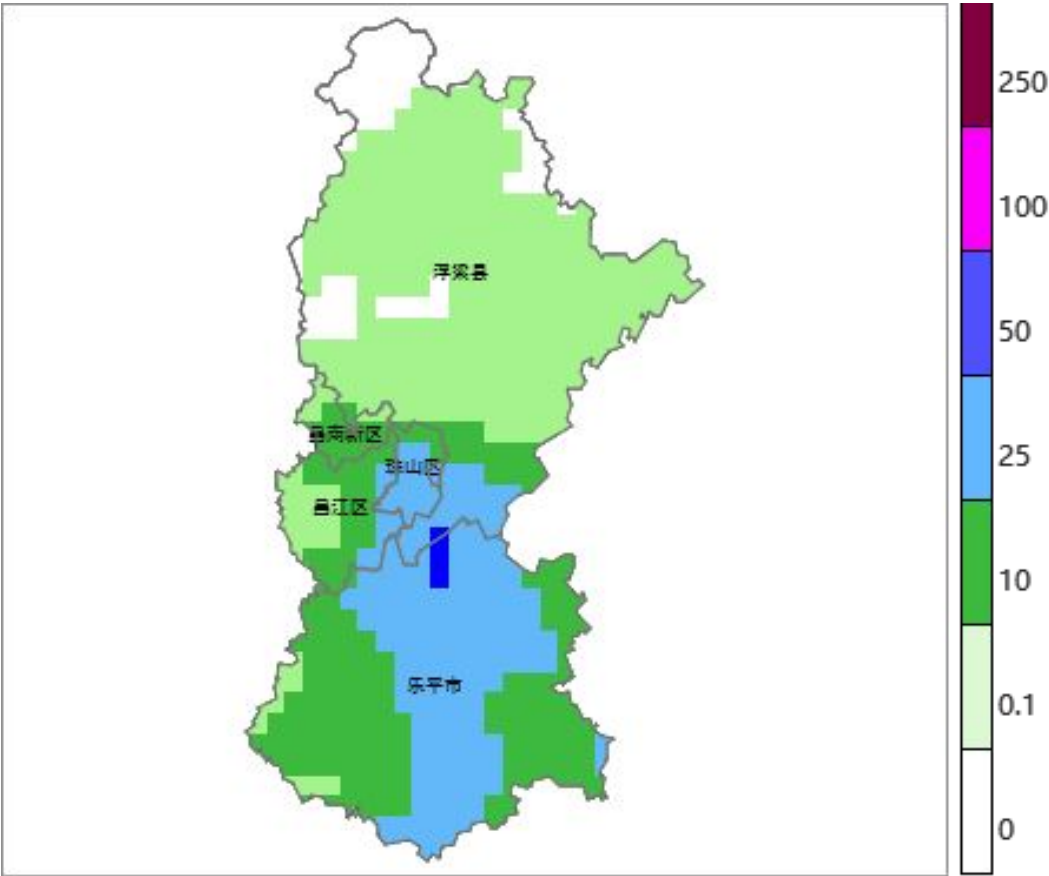
图 2 未来 3 小时(00:40-03:40)累计雨量预报图
